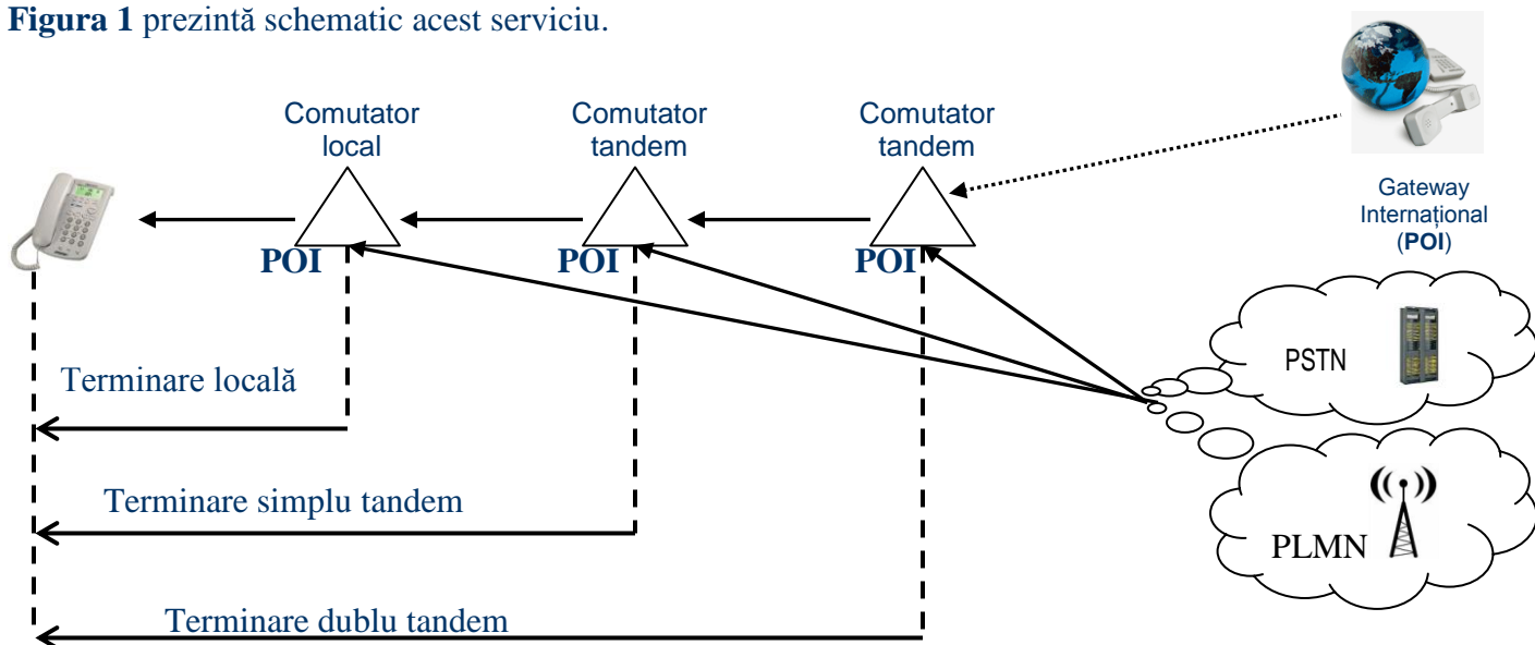
Figura 1: Serviciile de terminare de trafic în rețeaua publică telefonică fixă
